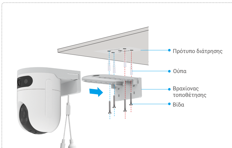
Εικ. 1 Τοποθέτηση στην οροφή
