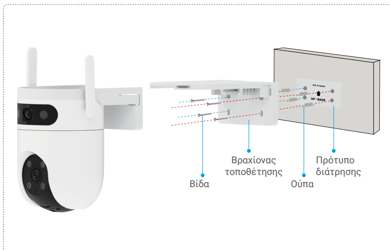
Εικ. 2 Τοποθέτηση στον τοίχο
